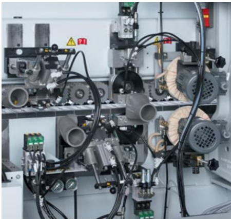
Raspadores de raio – Raspadores de cola Unidade de Polimento
