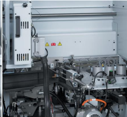
Alimentador de orla
