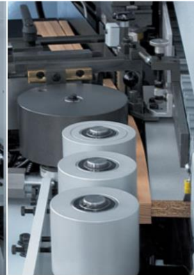
Zona de pressão
